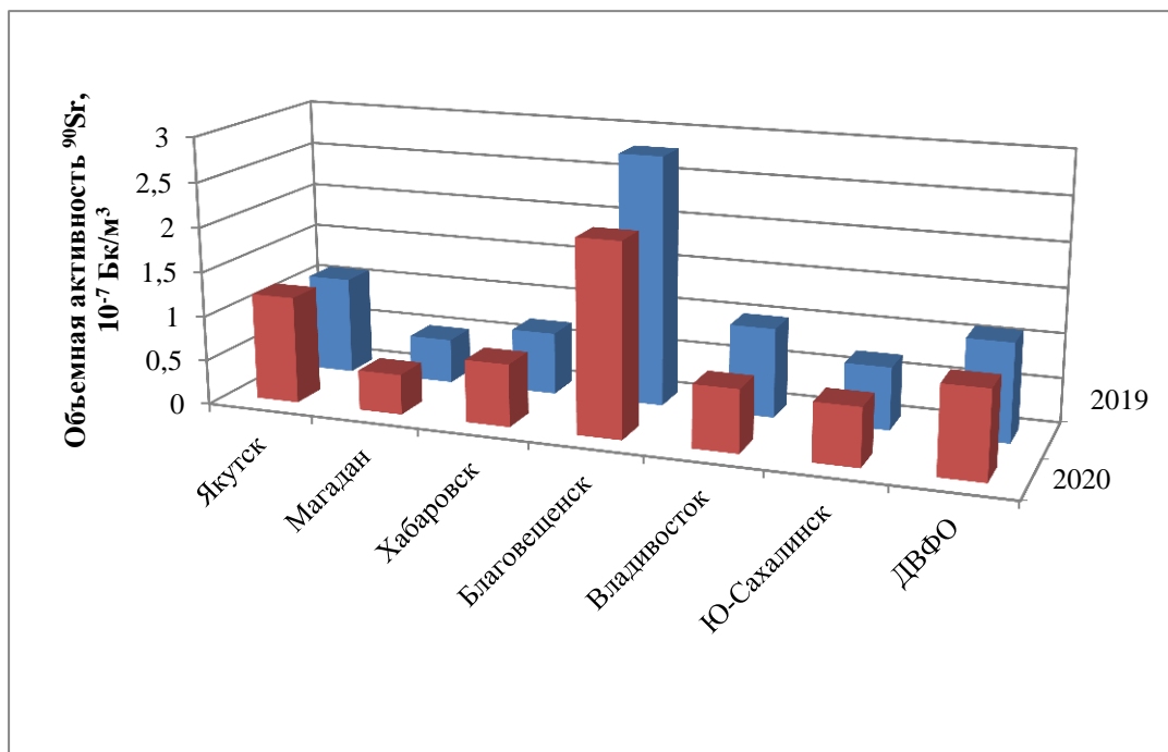
Рис. 2.39. Среднегодовая объемная активность 90 Sr в населенных пунктах ДВФО в 2019-2020 гг., 10 -7 Бк/м 3
