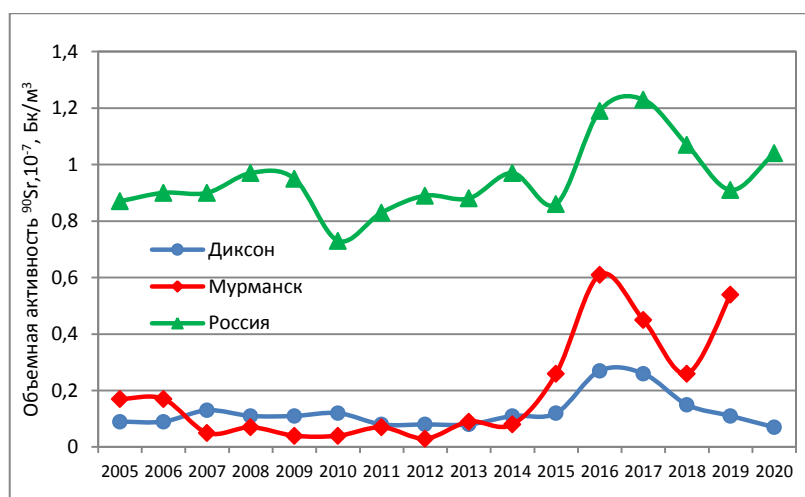
Рис. 4.55. Динамика объемной активности 90 Sr в воздухе на о. Диксоне, в Мурманске и средневзвешенной по России в 2005-2020 гг.
