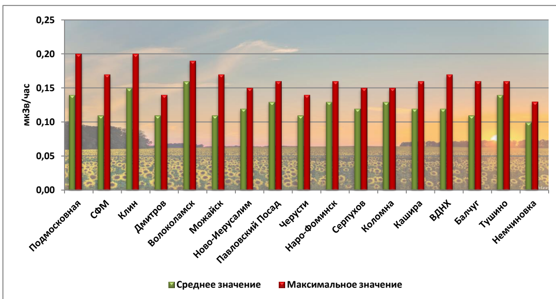
Рис. 4.12. Средние и максимальные значения мощности AMBIENTНОГО эквивалента дозы гамма-излучения (МАЭД) на станциях Московского региона в 2020 г.
