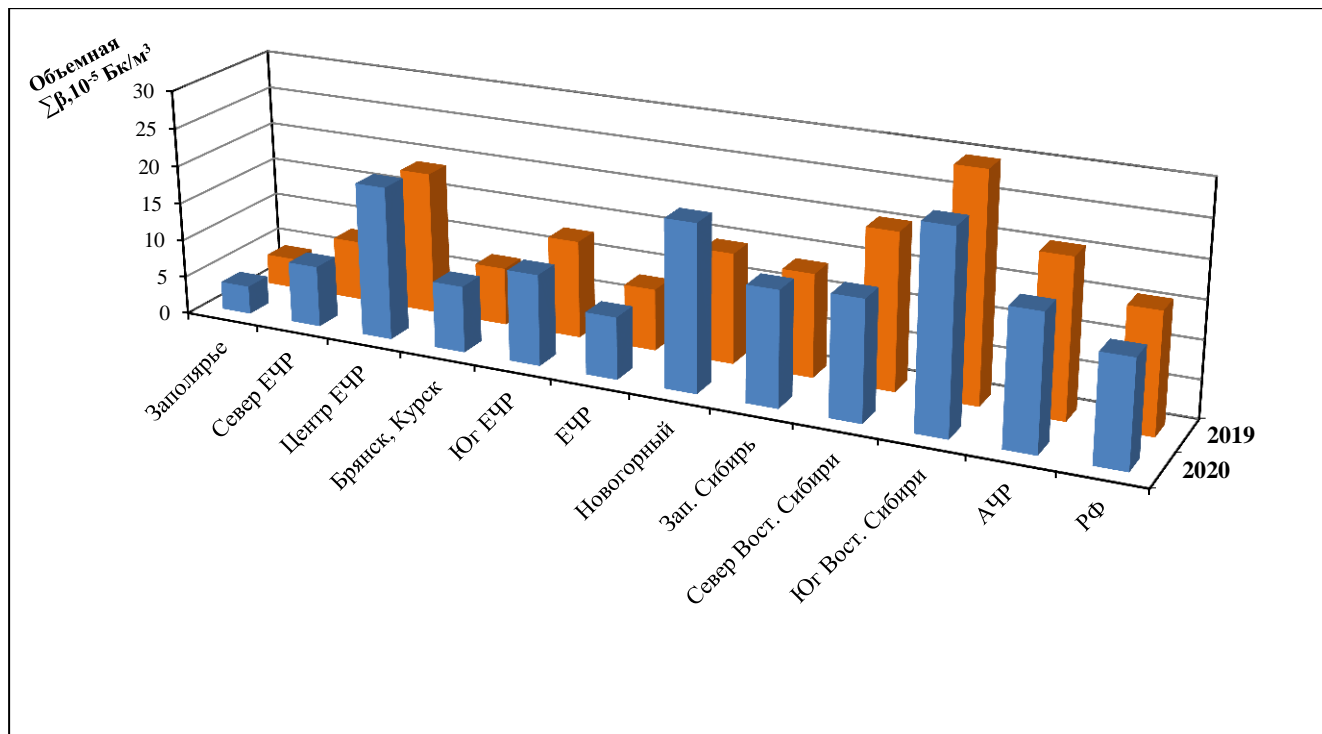
Рис. 2.36. Средние значения объемной \Sigma B в приземном слое атмосферы на территории РФ в 2019-2020 гг., 10^{-5} Бк/м 3
