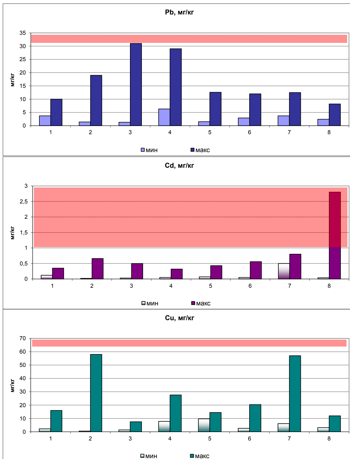
Рис. 2.33. Варьирование концентраций тяжелых металлов в почвах СКФМ за период 2010-2020 гг. СКФМ: 1 - НП Смоленское Поозерье, 2 - Приокско-Тerrasный БЗ, 3 - Воронежский БЗ, 4 - Кавказский БЗ, 5 - Астраханский БЗ, 6 - Волжско-Камский БЗ, 7 - Алтайский БЗ (Яйлю), 8 - Баргузинский БЗ.
