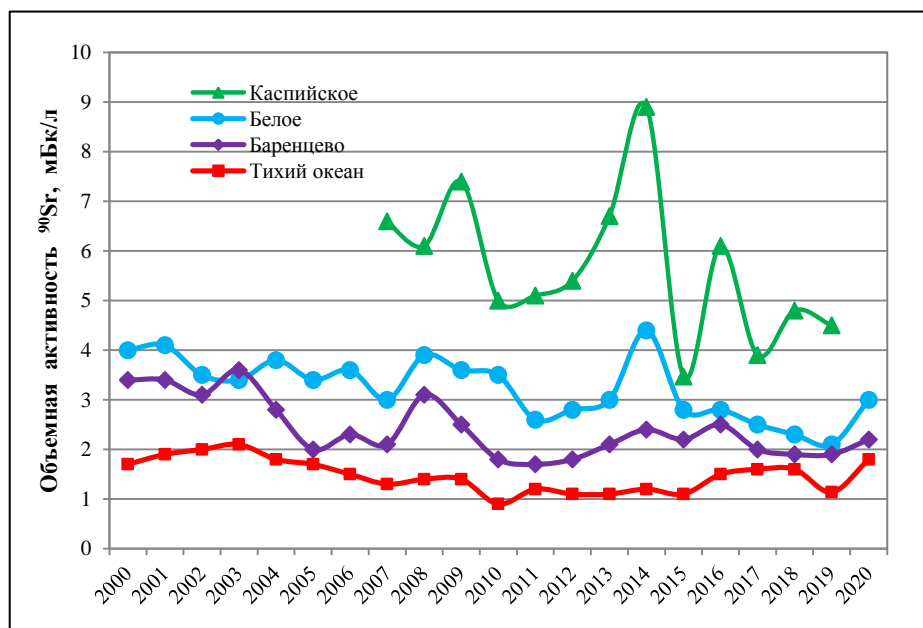
Рис. 4.56. Динамика объемной активности 90 Sr в прибрежных водах Белого и Баренцева морей в сравнении с водами Каспийского моря и Тихого океана вблизи восточного побережья Камчатки в 2000-2020 гг., мБк/л
