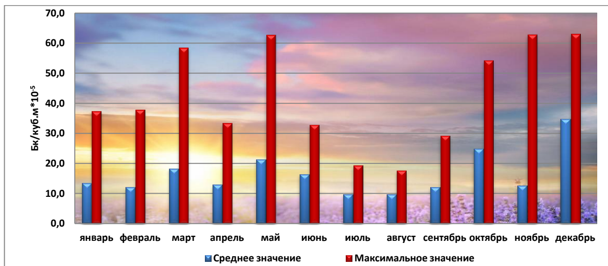
Рис. 4.10. Среднемесячные и максимальные значения объемной суммарной бета-активности радионуклидов в приземном слое атмосферы в 2020 г.
