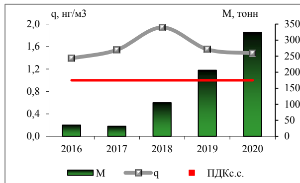
Рис. 3.13. Среднегодовые концентрации бенз(а)пирена (q, ng/m³) и выбросы от стационарных источников (M, тонн)
