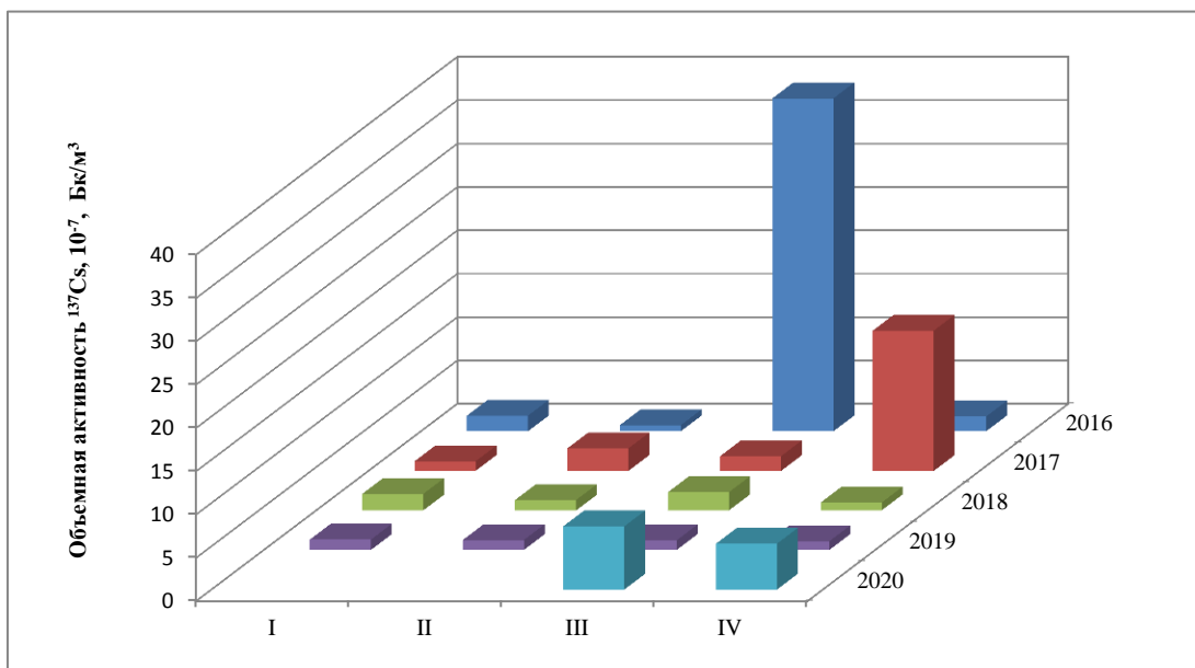
Рис. 4.54. Динамика средней за квартал величины объемной активности 137 Cs в воздухе в Мурманске в 2016-2020 гг.
