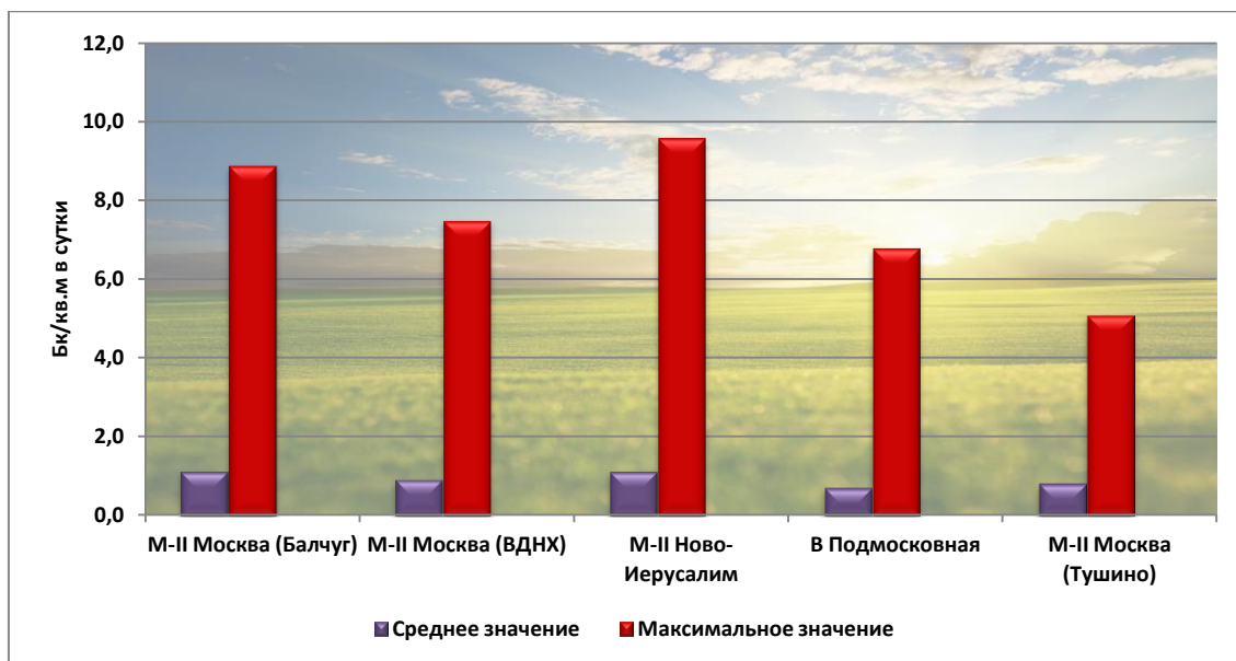
Рис. 4.11. Среднемесячные и максимальные суточные выпадения на станциях Московского региона в 2020 г.
