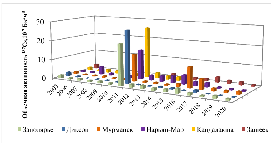
Рис. 4.53. Объемная активность 137 Cs в приземной атмосфере в пунктах наблюдения Сухопутных территорий Арктики и в среднем по Заполярью в 2005-2020 гг., 10 -7 Бк/м 3
